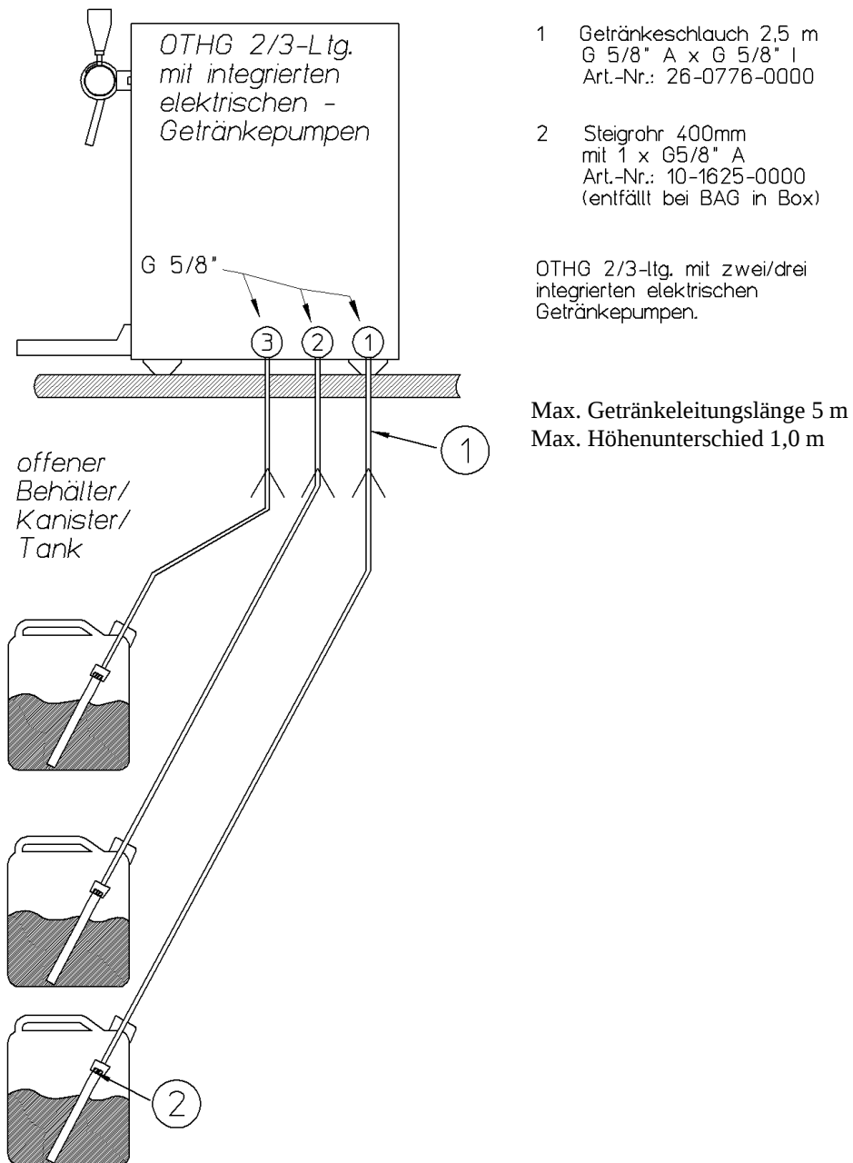
Prinzipskizze OTHG mit integrierter elektrischer Getränkepumpe
